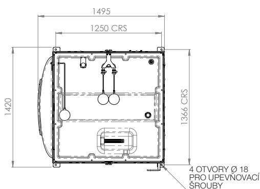
PŮDORYSY S VYNECHANÝM VÍKEM NÁDRŽE
